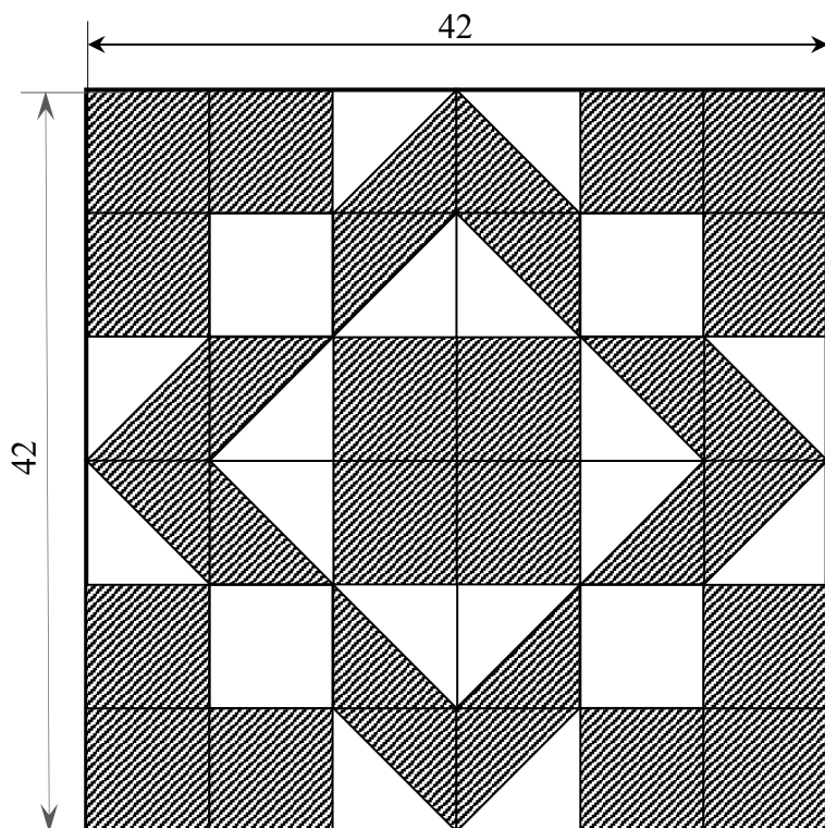
Рисунок 2 – Технический рисунок наволочки
